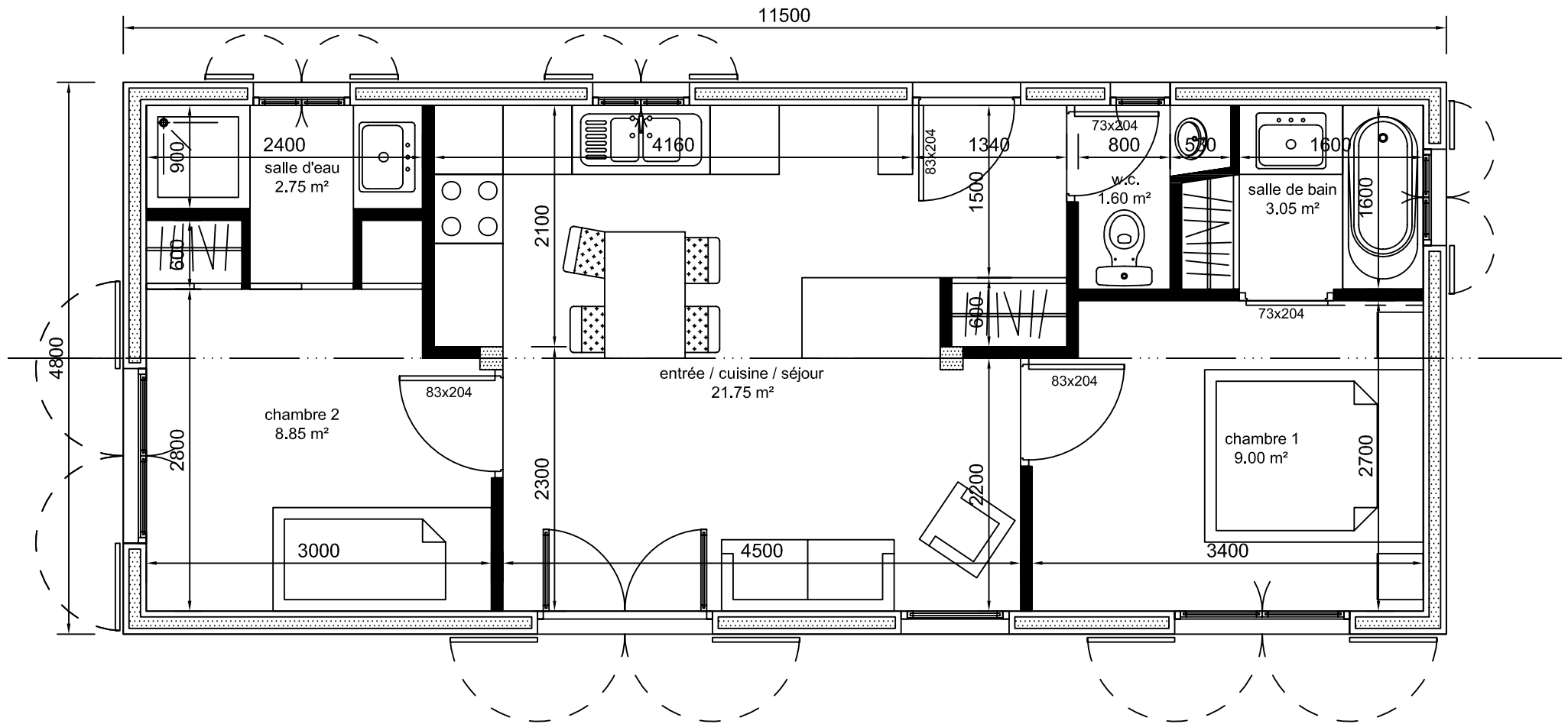
TECTOBOIS PYRENEEN I (11,5 x 4,8 mètres) Surface hors tout 55,20 m 2 Echelle 2 CM X M.
