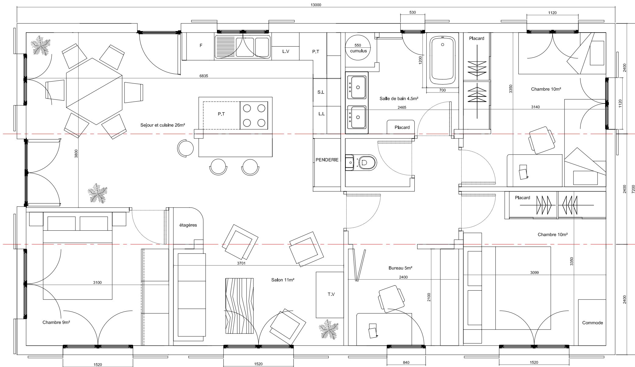
TECTO@73 3 VALLEES PILO (13 x 7.2 mètres) Surface hors tout 93,6 M² Echelle 1:50.
